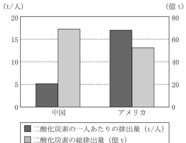
グラフⅢ 中国とアメリカにおける二酸化炭素の排出量 (2009 年)
